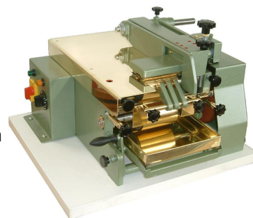
Zweiwalzen- Kantenanleimmaschine Mod. CORONEL 90 mm
