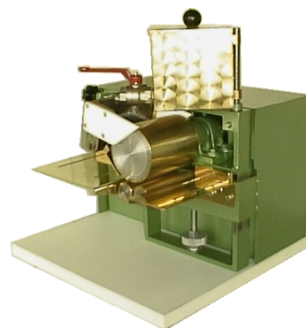
Kantenanleimmaschine mit Oberleimwerk Mod. MERCUR 120 mm
